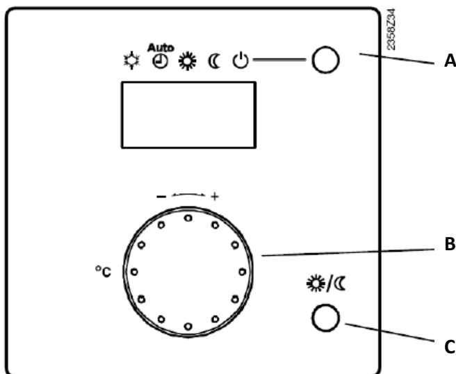
Figura 4.1 – Unità ambiente QAA55.110
