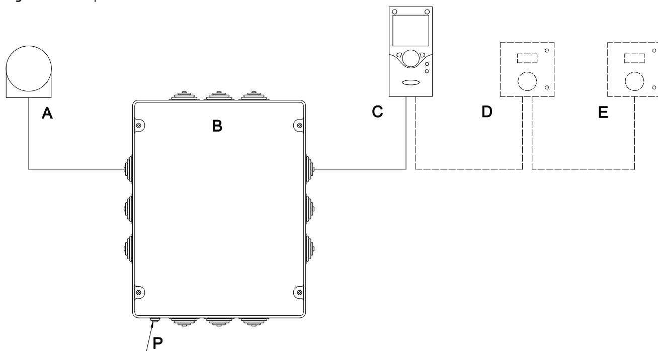
Figura 2.1 – Componenti del Controllore di Sistema K18
