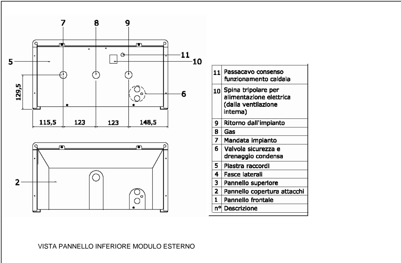
Figura 1 - VISTA MODULO ESTERNO
