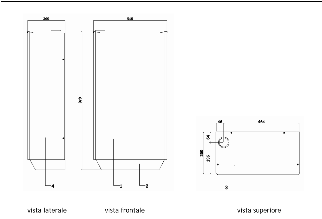
Figura 2 - DIMENSIONI MODULO ESTERNO
