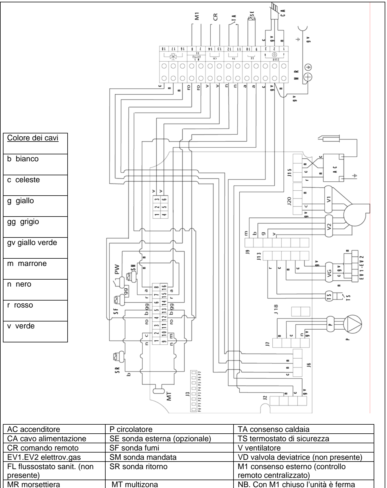
Figura 6 - SCHEMA COLLEGAMENTI SCHEDA ELETTRONICA MODULO ESTERNO
